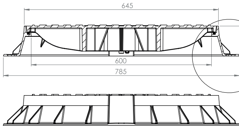
KESIT C-C ÖLÇEKLE 1 : 5
